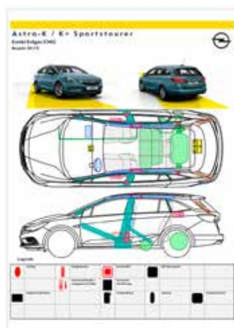
Rettungskarte/Rettungsdatenblatt
